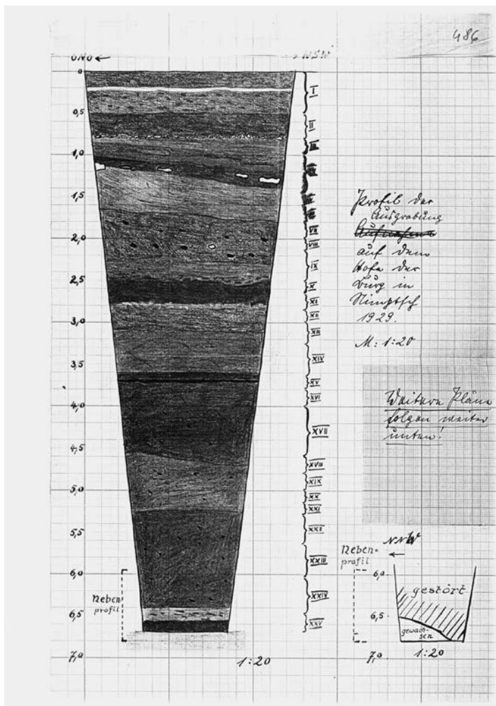
Abb. 35 Profilzeichnung von der Ausgrabung auf dem Burghof in Nimptsch 1929.
