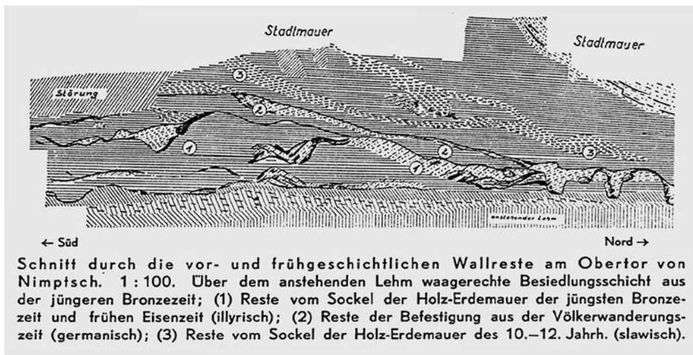
Abb. 39 Profilzeichnung zur Ausgrabung am Obertor in Nimptsch 1936, vermutlich aus Schnitt I (nach Petersen 1737 a, 17).
